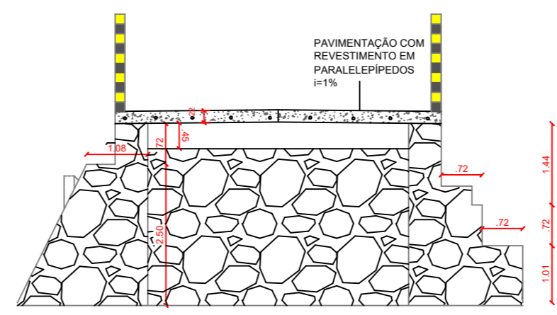
6 CORTE B-B S/ ESCALA
