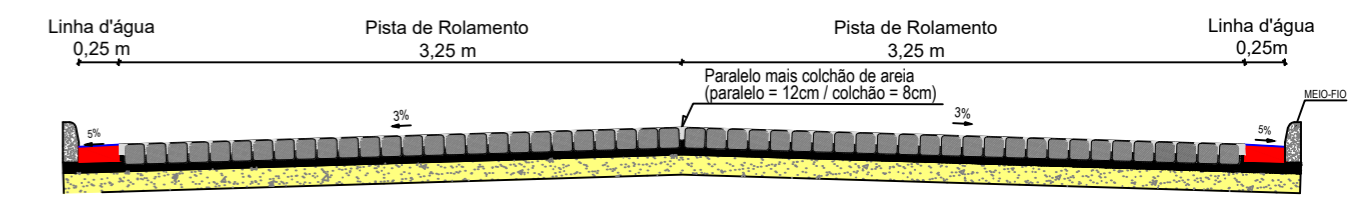
8 DETALHAMENTO - PAVIMENTAÇÃO S/ ESCALA
