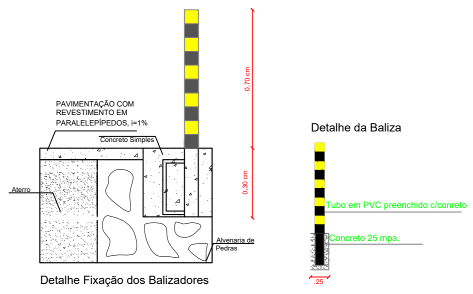
7 DETALHAMENTO - BALIZADORES S/ ESCALA
