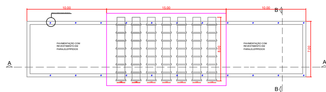
4 PASSAGEM MOLHADA - TRECHO 3 1:250
