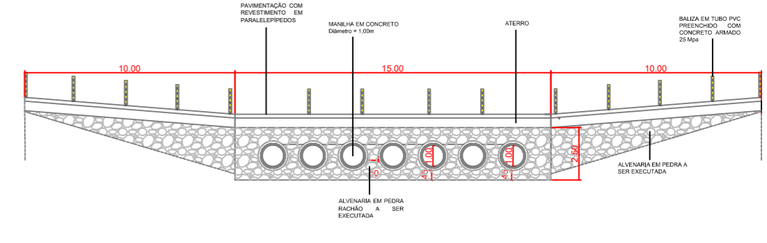
5 CORTE A-A 1:250
